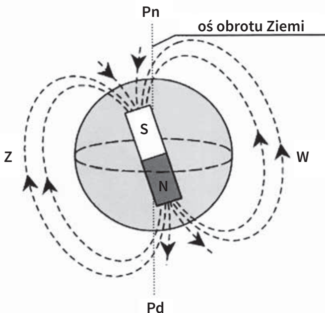
Rysunek 13. Obraz pola magnetycznego Ziemi.
