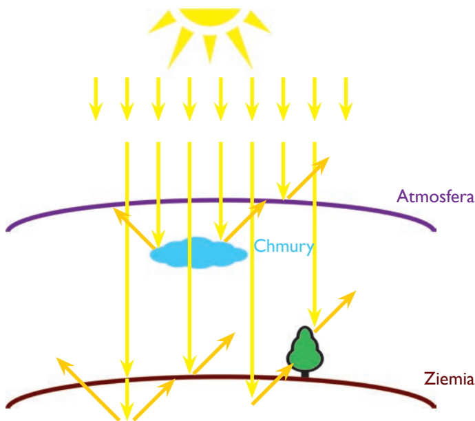
Rys. 2a. Zasoby spływającej energii słonecznej znajdują się nie tylko w powietrzu, ale i również trafiają w: skały, wodę (strumyki, rzeki), drzewa i inne rośliny
